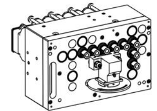
Cabezal B 8 brocas verticales, de las cuales 6 en eje X y 2 en eje Y, y una sierra en eje X. Boring Head B 8 vertical spindles, 6 on X axis and 2 on Y axis, and a saw on X axis.
