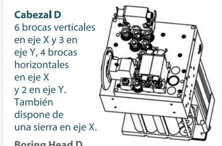
Cabezal D 6 brocas verticales en eje X y 3 en eje Y, 4 brocas horizontales en eje X y 2 en eje Y. También dispone de una sierra en eje X. Boring Head D 6 vertical spindles on X axis and 3 on Y axis, 4 horizontal spindles on X axis and 2 on Y axis. Also a saw on X axis.
